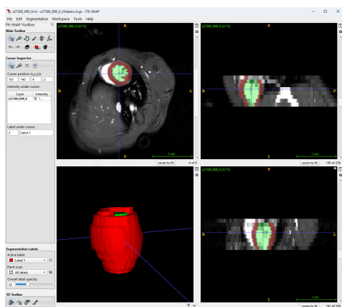
ITK-SNAP
